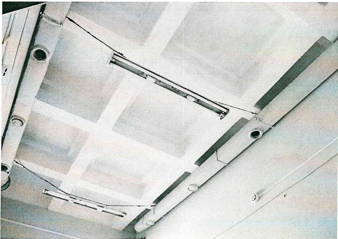
Видовая точка № 8. Монолитное железобетонное кессонное перекрытие в помещении реконструированной части здания (1963 г.).
